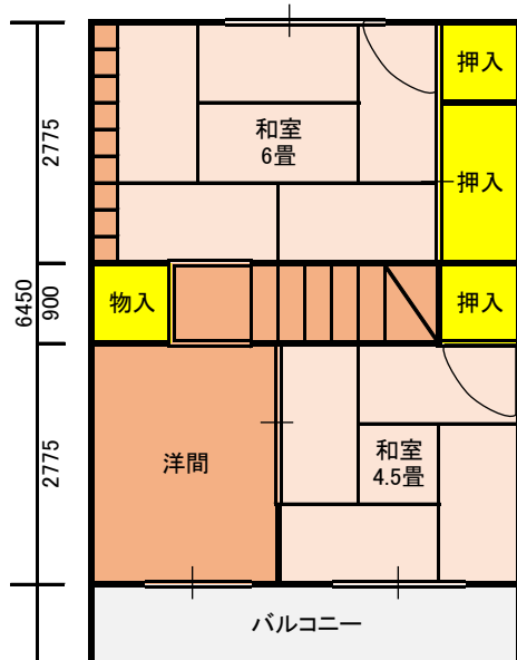
4DKタイプ
