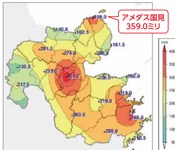
図1：2024年8月29日 日降水量分布図
