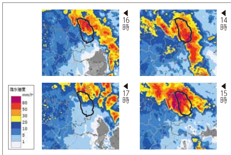
図2：2024年8月29日 雨雲の動き
