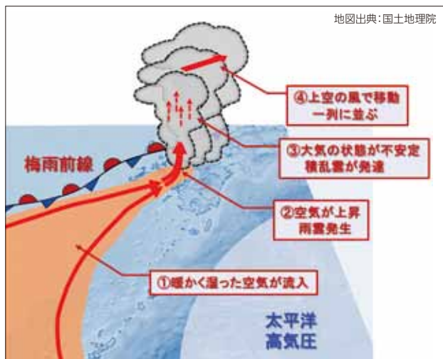
図3：梅雨時期の大雨発生メカニズム
