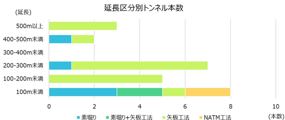
図-2.9 延長区分別トンネル本数
