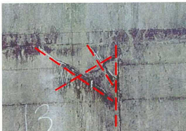
ブロック化したひび割れの例の図と写真
