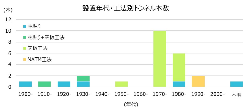
図-2.7 設置年代・工法別トンネル本数
