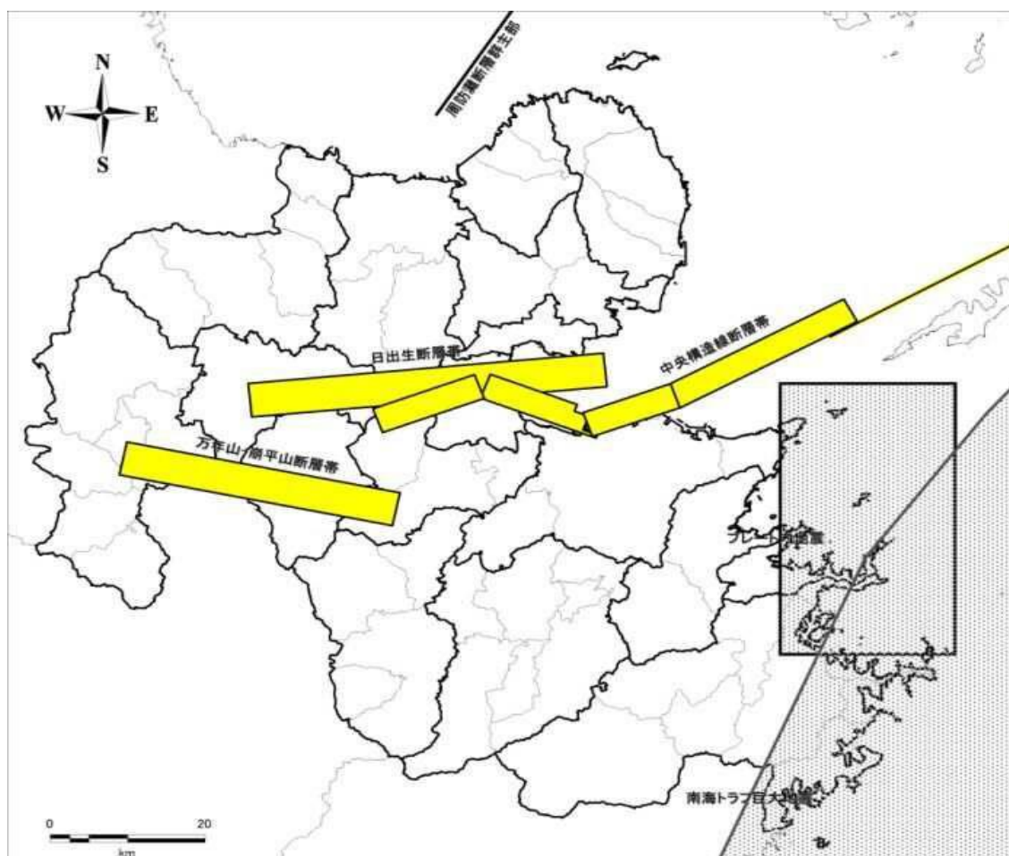
地震位置図
